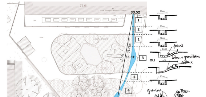
Schéma et coupes de principes sur la rivière pédagogique | © CAUE de Paris
