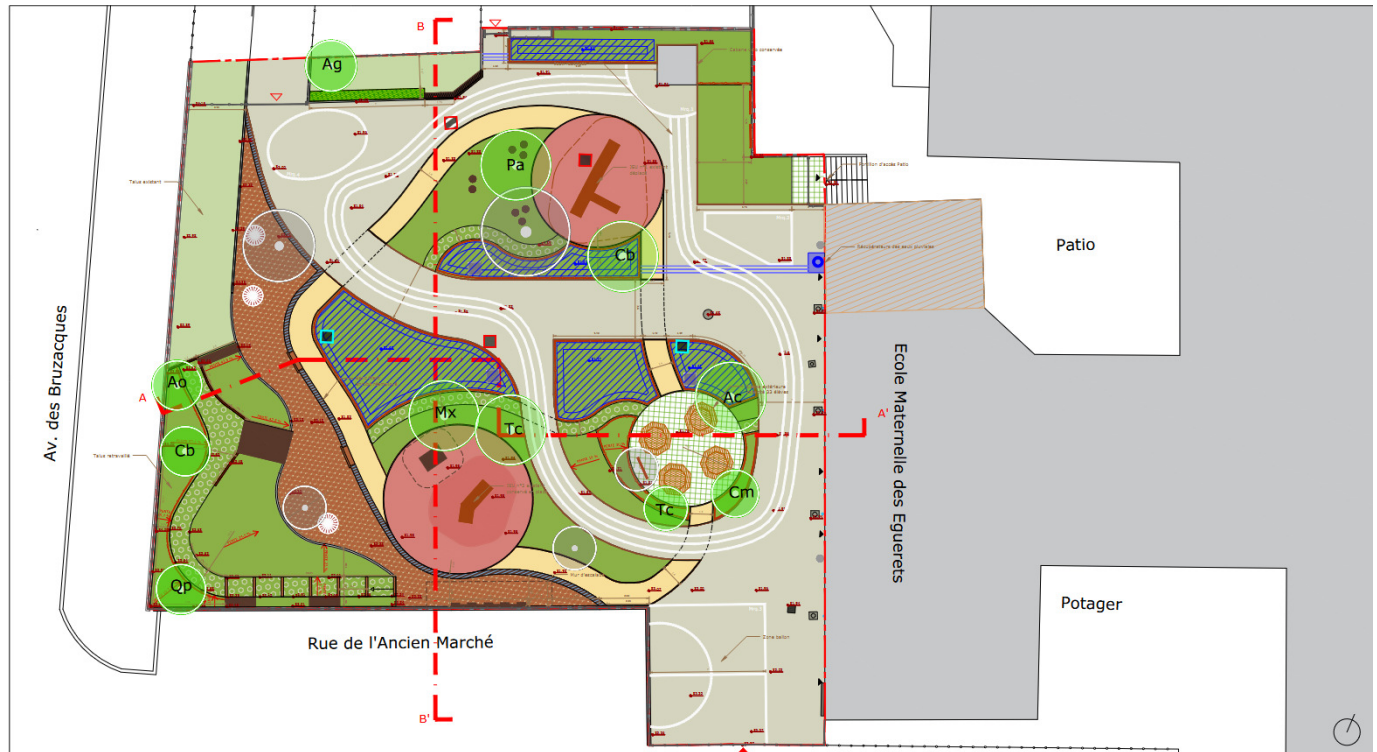
Plan phase pro de la Cour des Eguérets | © Urban water
